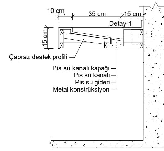
B-B KESİTİ
