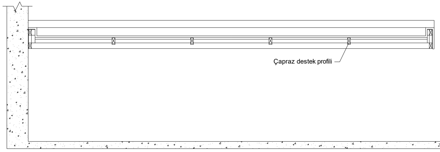
A-A KESİTİ
