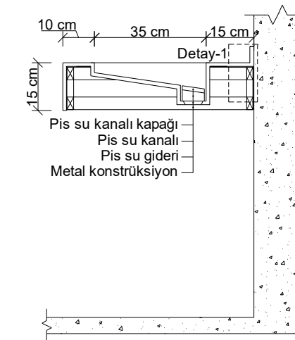
B-B KESİTİ
