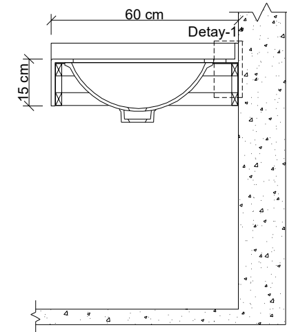
B-B KESİTİ
