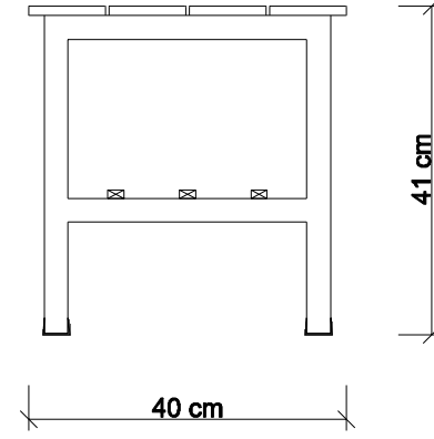
Yandan Görünüş
