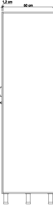
YAN GÖRÜNÜŞ
